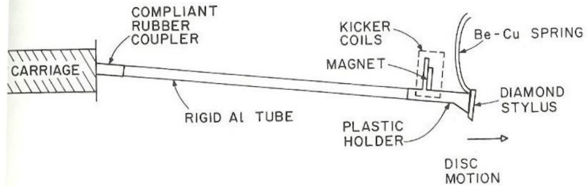
Fig. 4—Stylus arm.
